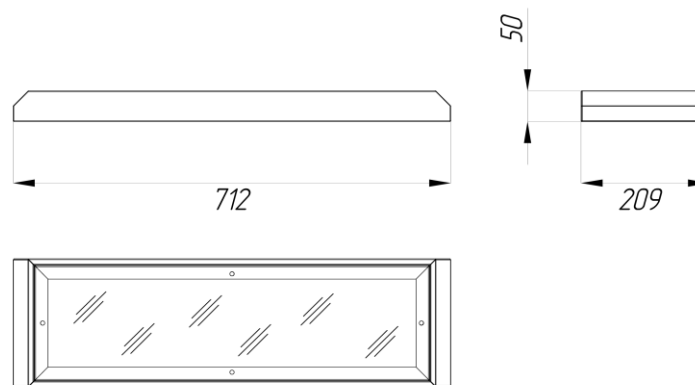
Рисунок 1. Габаритные размеры светильника ДПО20-16
