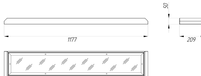
Рисунок 2. Габаритные размеры светильников ДПО20-32, ДПО20-37, ДПО20-64
