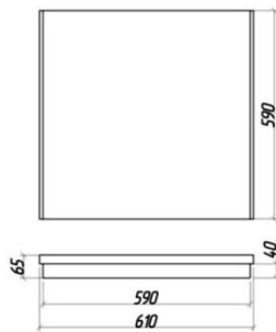
Рисунок 3 – Габаритные размеры светильников серии Грильято.
