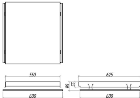
Рисунок 4 – Габаритные размеры светильников серии Экофон.
