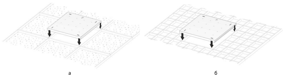
Рисунок 7 - Установка светильника Geniled серии Офис, ЛПО (а), серии Грильято (б) на подвесную конструкцию.
