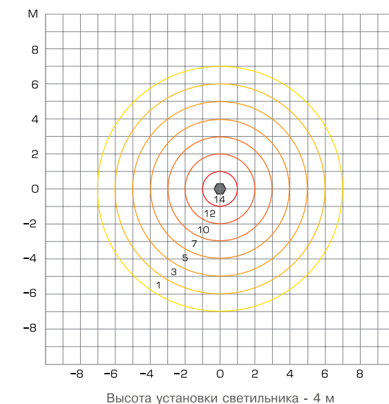
Диаграмма освещенности для светильника «Ораниенбаум» 100 Вт с прозрачным стеклом, Ix
