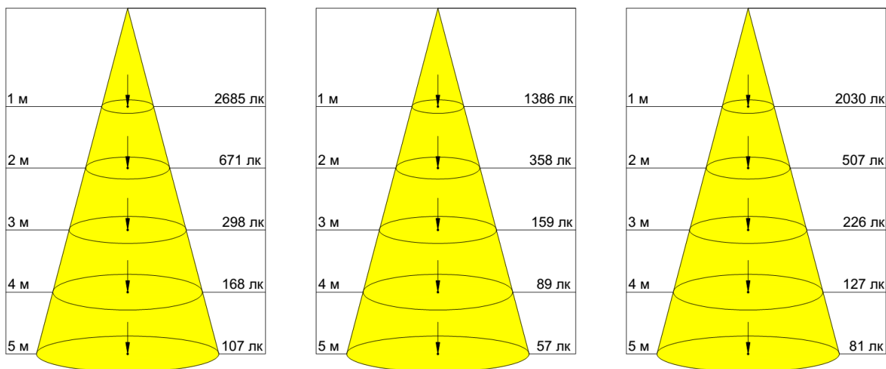
Микропризма 90°
