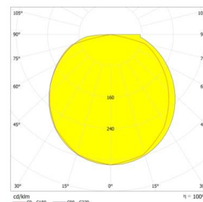
Рисунок 3 – Световое распределение.
