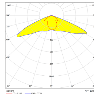
Рисунок 2 – Световое распределение светильника Geniled Консоль 150W.
