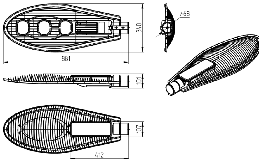
Рисунок 3 – Габаритный чертеж светильника Geniled Консоль 150W.
